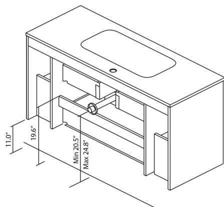
1 Door - 2 Drawers - 1 Door
